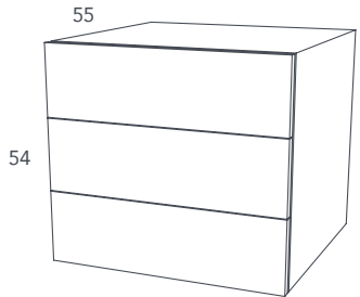
cajonera 3 cajones • Fondo 55 cm
