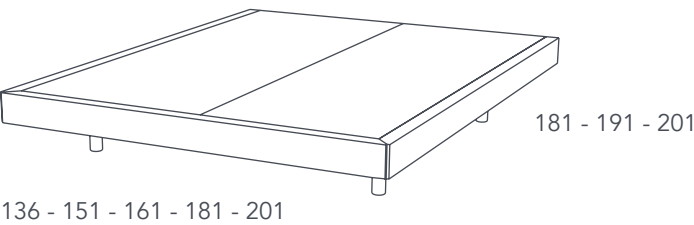
base Meet de 12 cm • Alto total 30 cm, grueso 4 cm sin patas decorativas en los extremos
