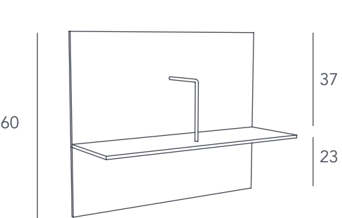
cabezal ART. Lateral opción 2- liso colgado • Altura 60 cm
