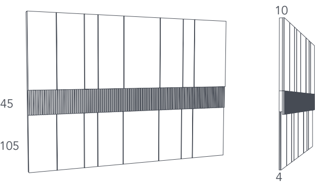
Listones 2x2 medidas fijas.
